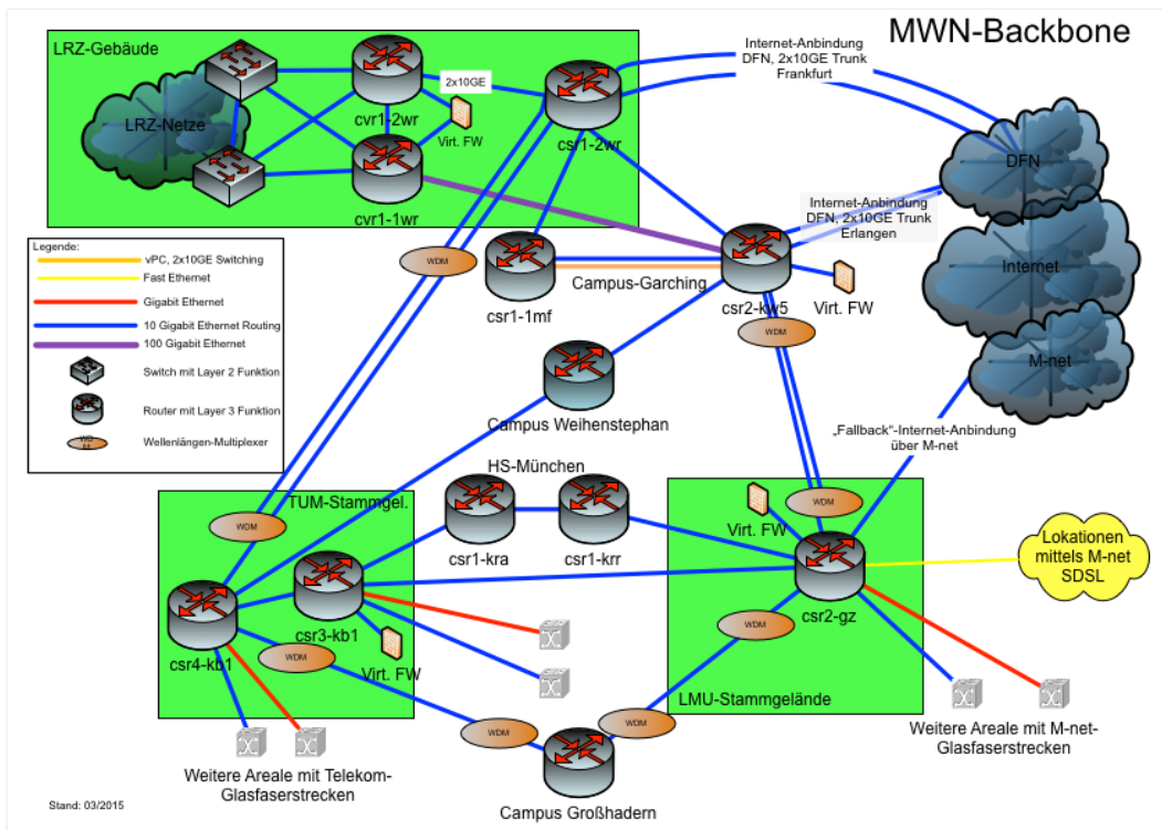
Abbildung 6: Backbonenetz des MWN
