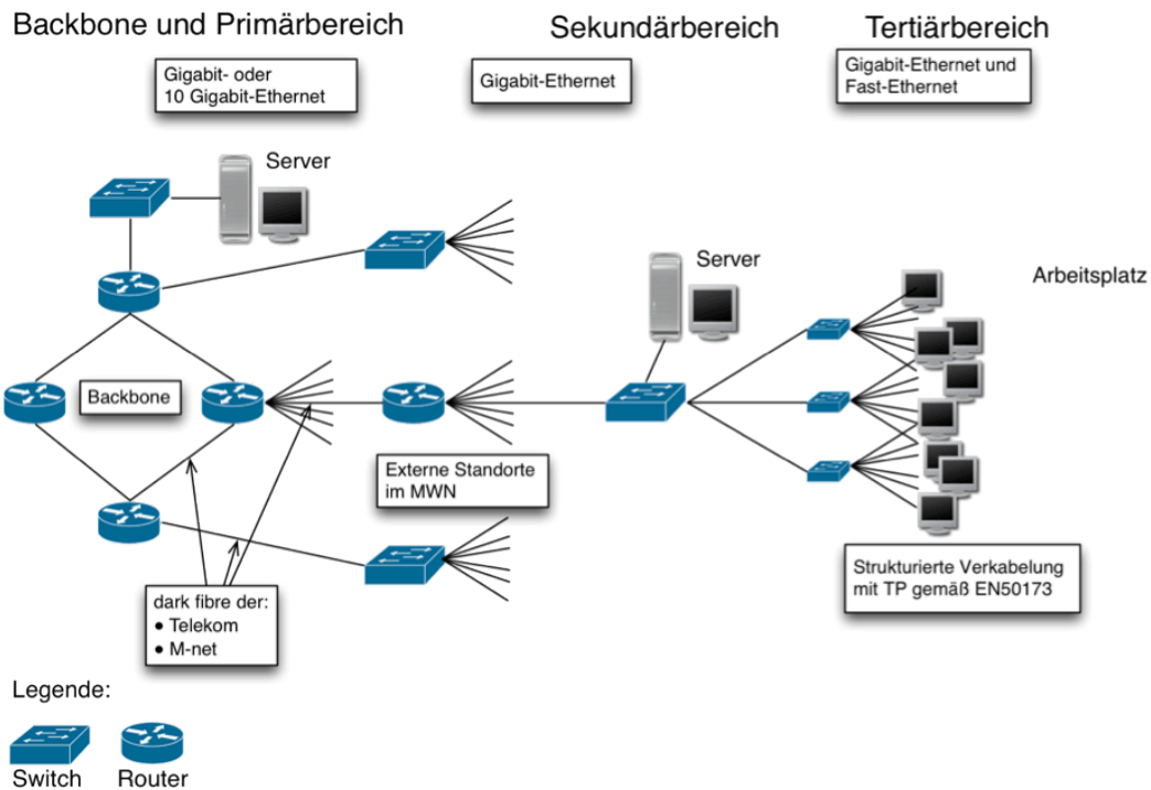
Abbildung 7: Schematische Verkabelungsstruktur
